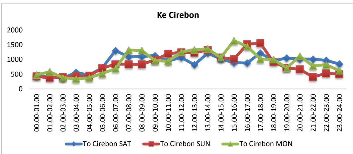
Gambar 2-38 Distribusi volume lalu lintas pada rute menuju ke Cirebon di ruas jalan Pantura, berdekatan dengan Jalan Akses 1, mulai hari Sabtu hingga Senin.
