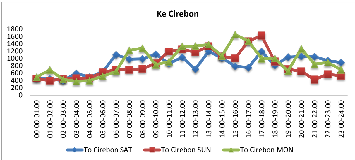
Gambar 2-40 Satuan Mobil Penumpang (SMP) untuk lalu lintas menuju ke Cirebon pada ruas jalan Pantura, yang berdekatan dengan Akses Jalan 1.
