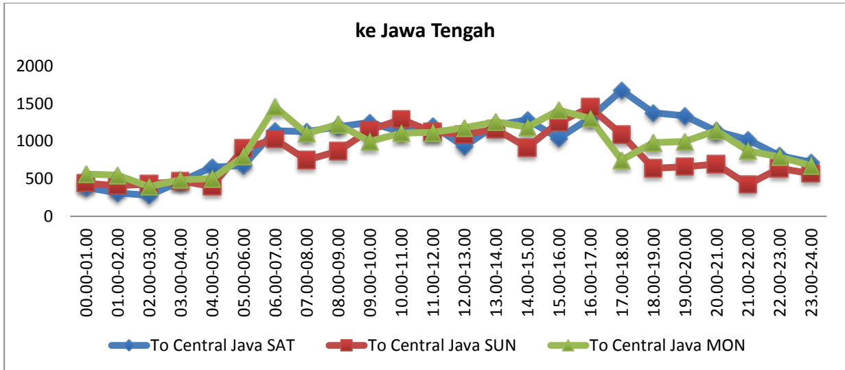
Gambar 2-37 Distribusi volume lalu lintas pada rute menuju ke Jawa Tengah di ruas jalan Pantura, berdekatan dengan Jalan Akses 1, mulai hari Sabtu hingga Senin.
