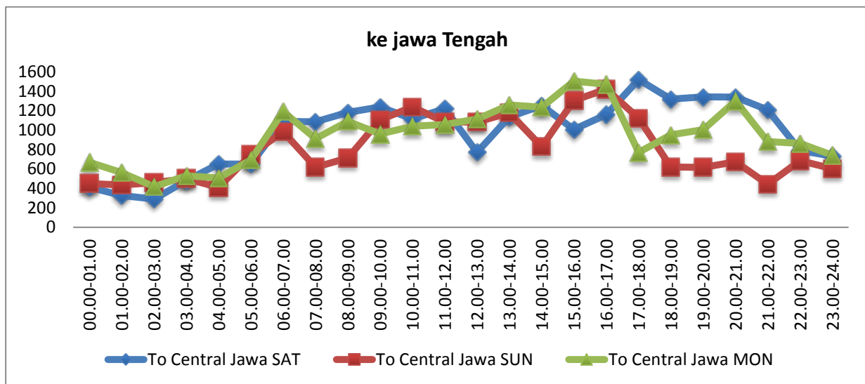
Gambar 2-39 Mobil Penumpang (SMP) untuk lalu lintas menuju ke Jawa Tengah di ruas jalan Pantura yang berdekatan dengan Jalan Akses 1.
