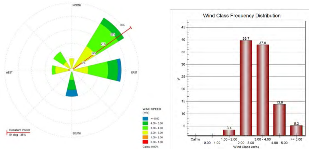
Gambar 2-5 Windrose ( blowing from ) sepuluh tahunan di Kabupaten Cirebon.
