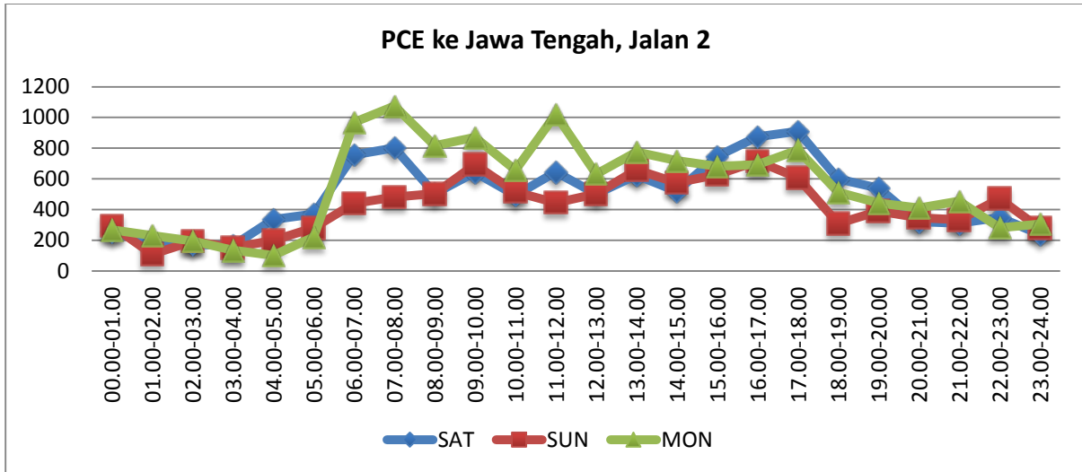
Gambar 2-46 Satuan Mobil Penumpang (SMP) untuk lalu lintas menuju ke Cirebon pada ruas jalan Pantura, yang berdekatan dengan Jalan Akses 2.
