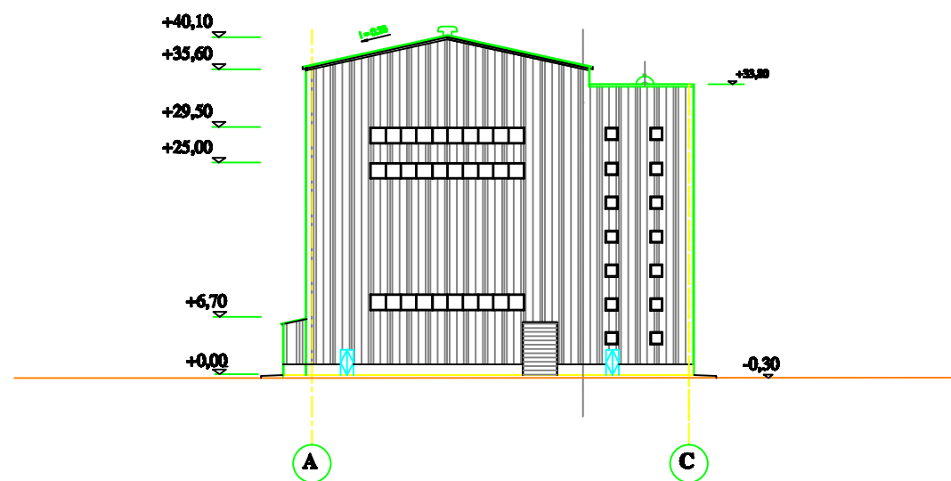
MẶT ĐỨNG TRỤC A-C ELEVATION AXIS A-C
