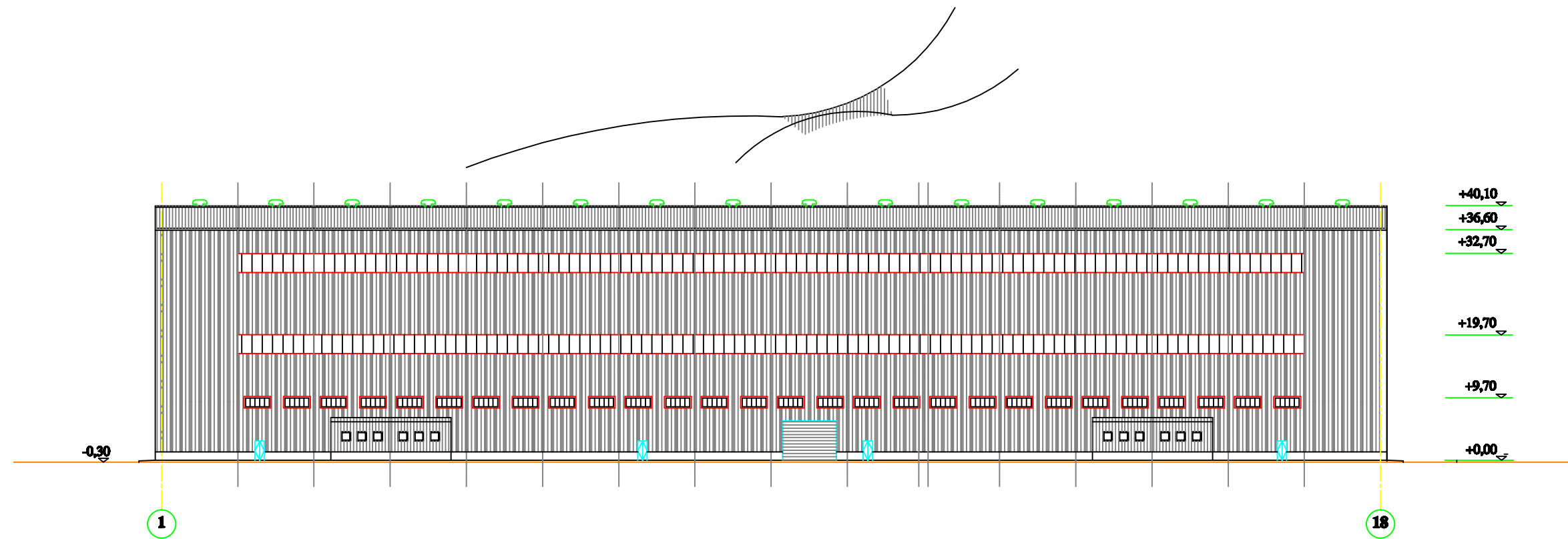
MẶT ĐỨNG TRỤC 1 - 18 FRONT ELEVATION AXIS 1 - 18
