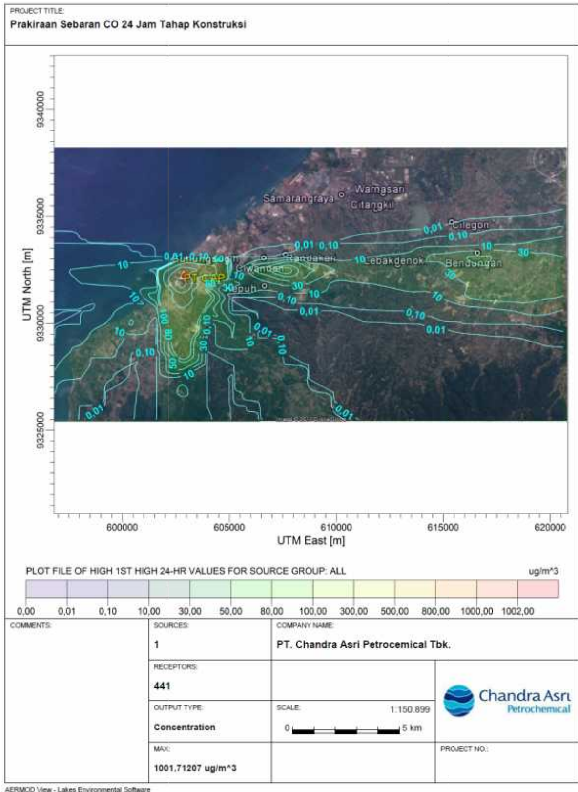
Gambar 3.1. Prediksi Sebaran CO 24 Jam Tahap Konstruksi
