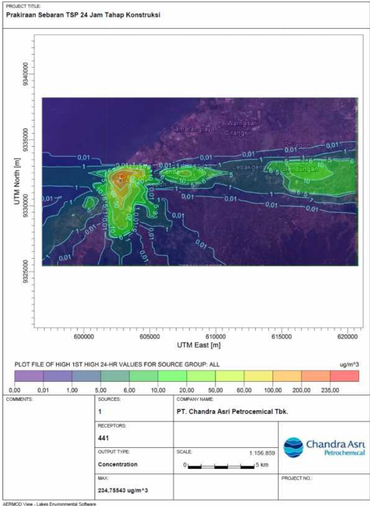
Gambar 3.4. Prediksi Sebaran TSP 24 Jam Tahap Konstruksi
