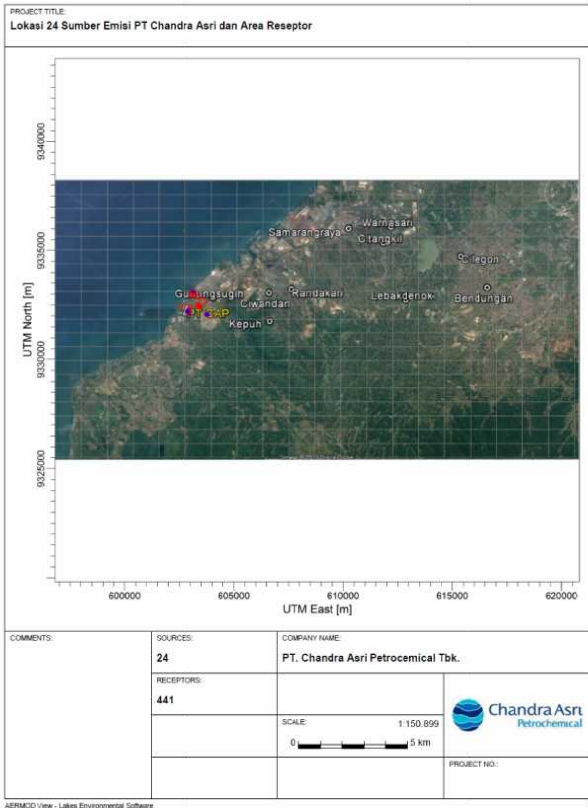
Gambar 3.6. Lokasi Sumber Titik PT Chandra Asri
