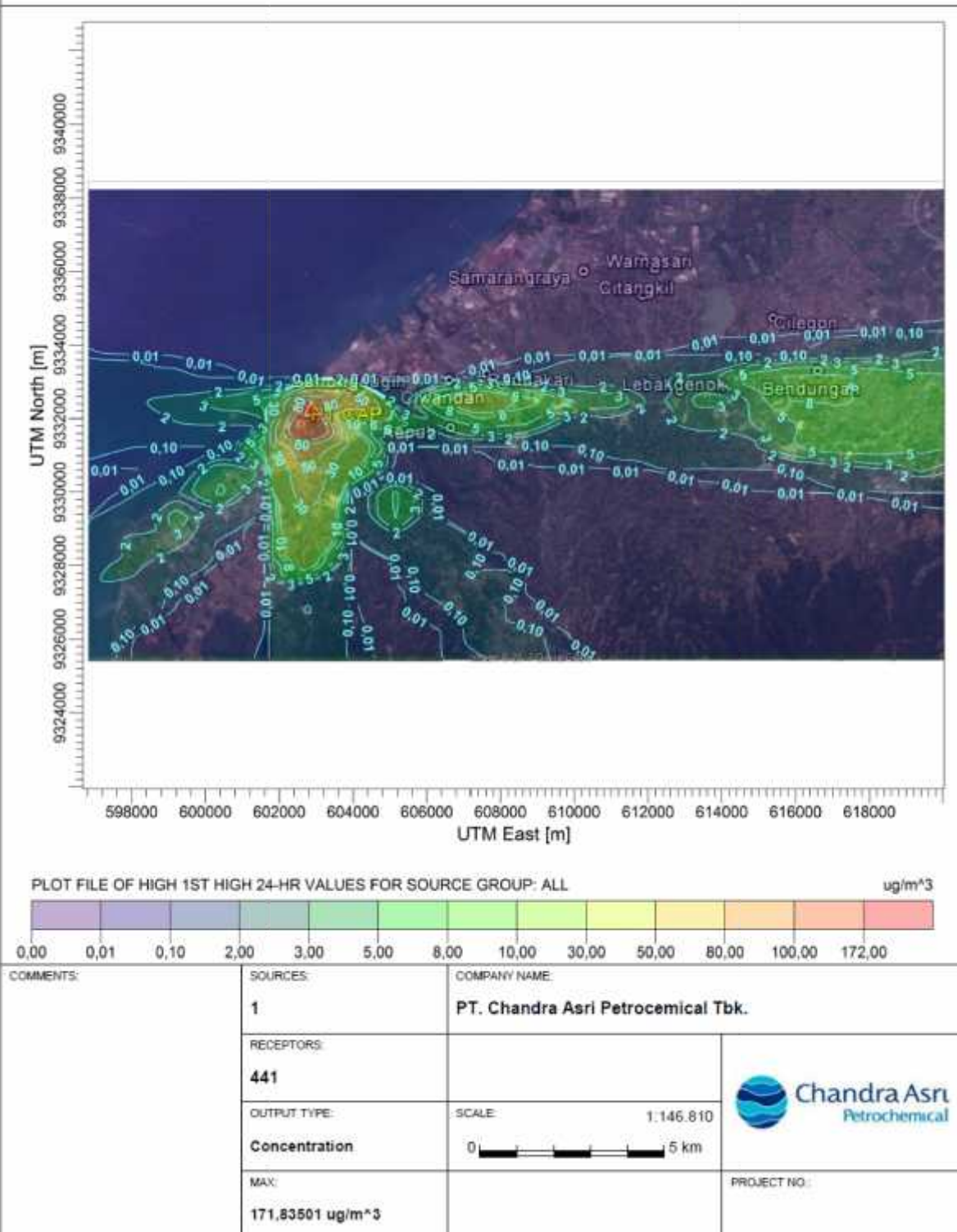
Gambar 3.5. Prediksi Sebaran PM10 24 Jam Tahap Konstruksi
