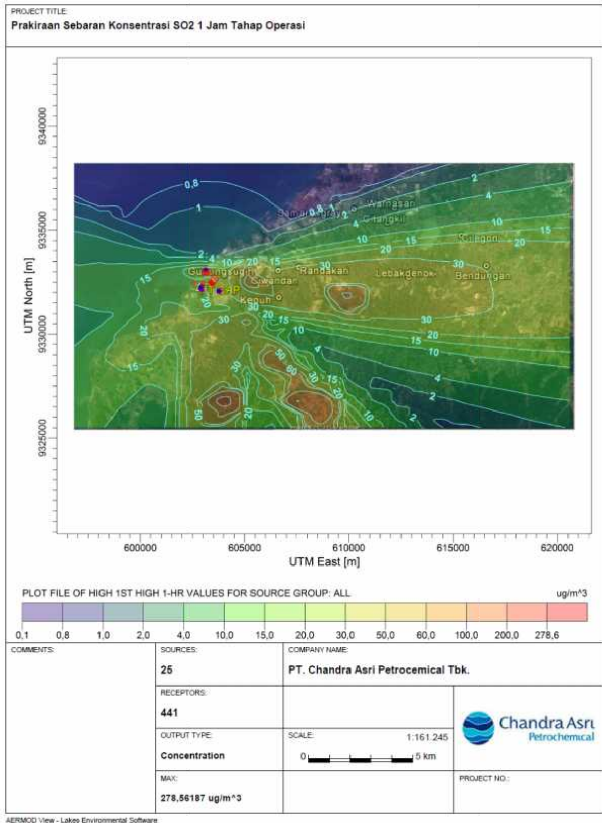
Gambar 3.12. Prakiraan Sebaran Konsentrasi SO 2 Rata-rata 1 jam (μg/m 3 ) dari Kegiatan Operasional PT Chandra Asri
