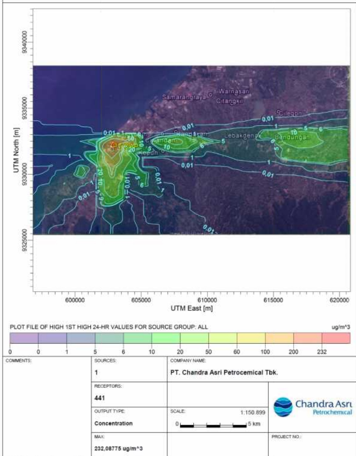
Gambar 3.3. Prediksi Sebaran SO 2 24 Jam Tahap Konstruksi
